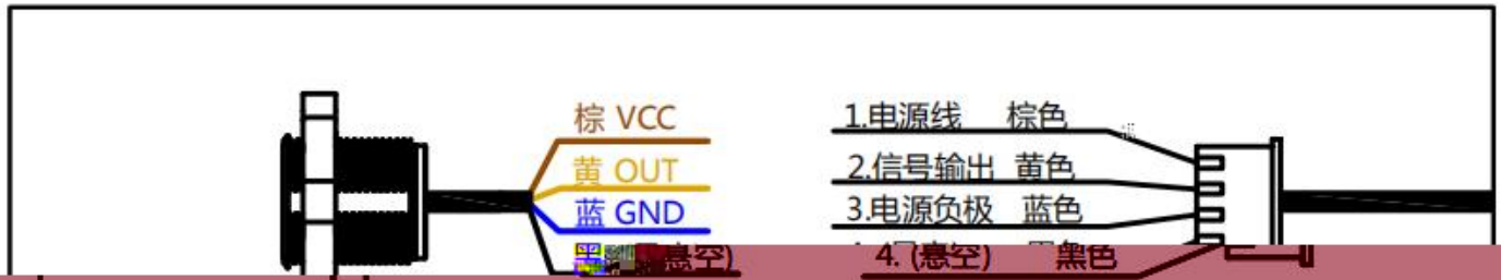
接线端口定义
